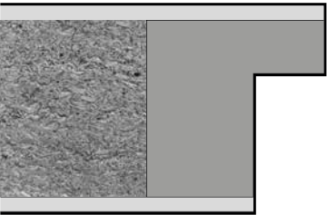
ECKIGE KANTE – EC CHANT CARRÉE – EC
